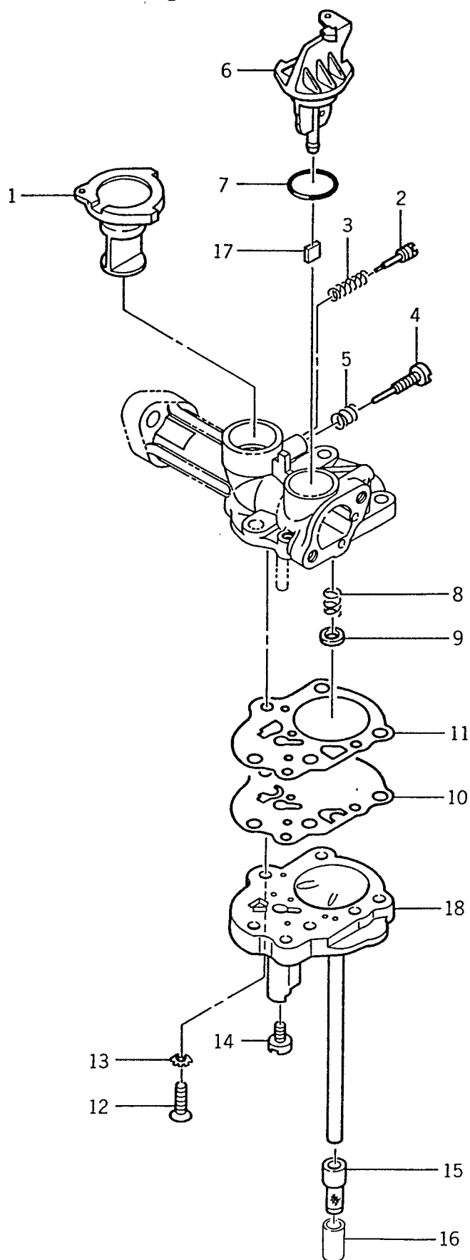
Fig. C-1 CARBURETOR
