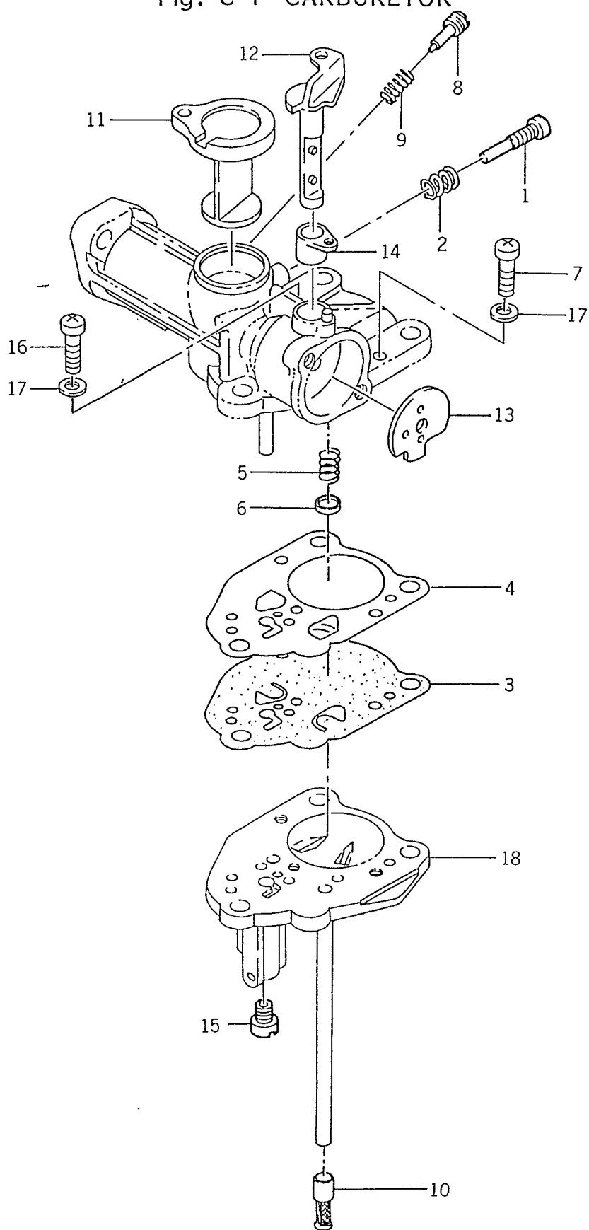
Fig. C-1 CARBURETOR
