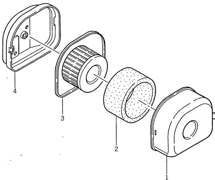
Fig. A-1 AIR CLEANER
