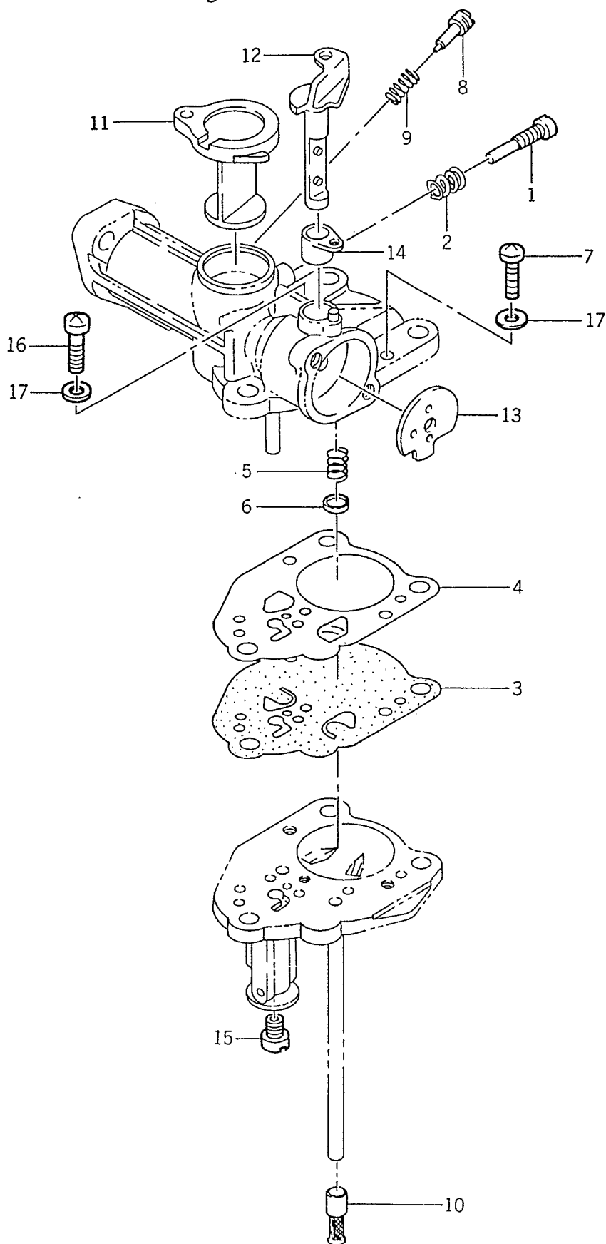
Fig. C-1 CARBURETOR
